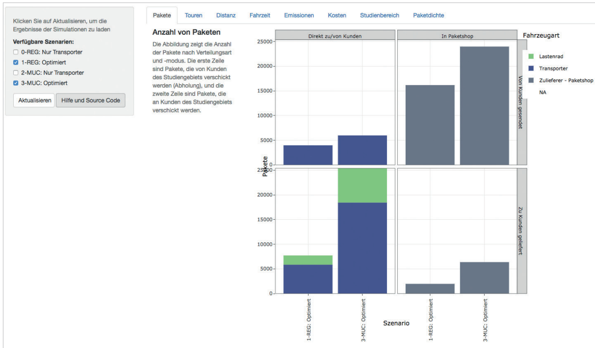
Abbildung 24: Visualisierungswerkzeug - Simulationsmodell - Pakete
